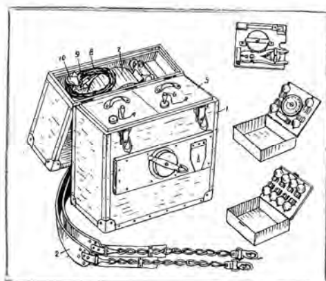
Kenttäpuhelin P-1-16 3 kpl
